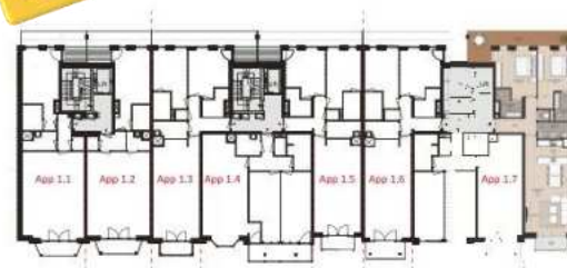
Overzicht 1 e verdieping
